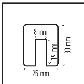
Élvédő profil E8 #1127-130
