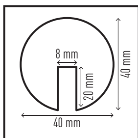
Élvédő profil E8R #1126-130
