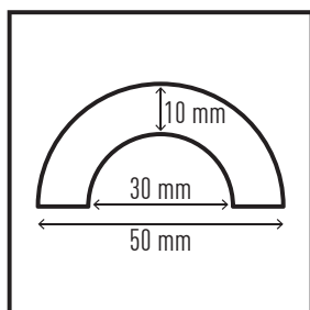
Csővédő profil P30 #1115-130
