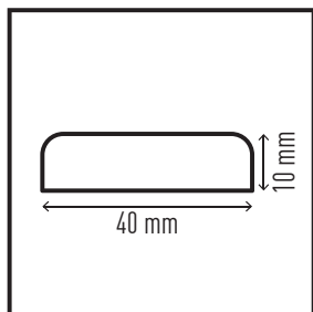
Felületvédő profil S10 #1107-130
