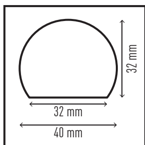
Felületvédő profil S32R #1109-130
